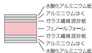
<フェノバボードフネンSR> (両面不燃仕様)
